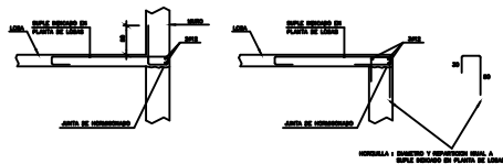
DETALLE ALTERNATIVO SUPLES EN MUROS SECCION 1-1
